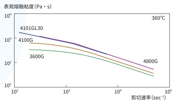
图4-2-2 表观熔融粘度的剪切速率依赖性
