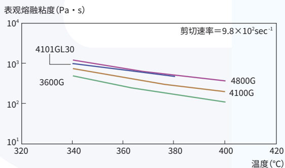
图4-2-1 表观熔融粘度的树脂温度依赖性
