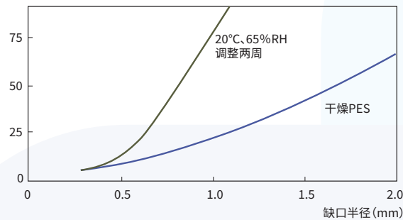
图3-2-5 冲击强度的缺口半径依赖性20℃(4800G) 简支梁冲击强度(kJ/m 2 )
