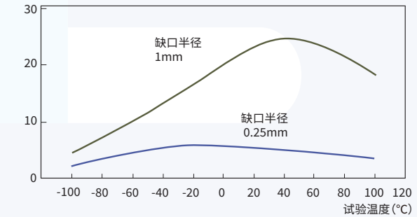
图3-2-6 冲击强度的温度依赖性(4800G) 简支梁冲击强度(kJ/m 2 )
