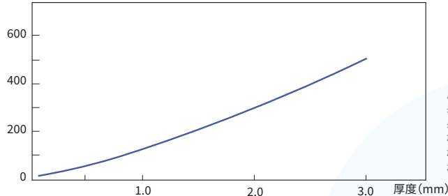
图4-2-6 BARFLOW长的厚度依赖性(4100G)
