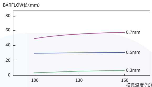
图4-2-17 模具温度依赖性(3601GL20)
