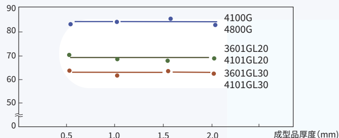
图3-2-9 成型品厚度与结合线位置拉伸强度的关系
