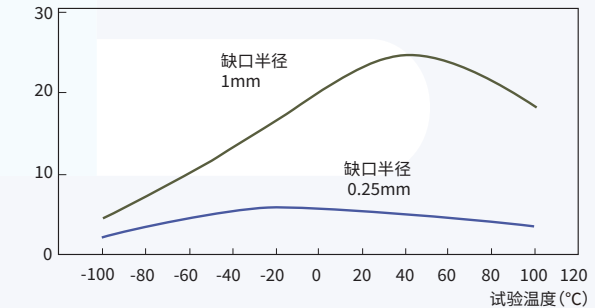
图3-2-6 冲击强度的温度依赖性(4800G) 简支梁冲击强度(kJ/m²)
