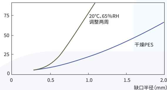
图3-2-5 冲击强度的缺口半径依赖性20℃(4800G) 简支梁冲击强度(kJ/m²)
