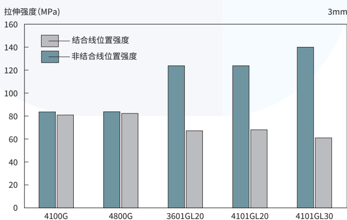
图3-2-7 拉伸强度
