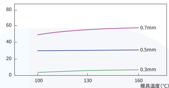
图4-2-17 模具温度依赖性(3601GL20)
