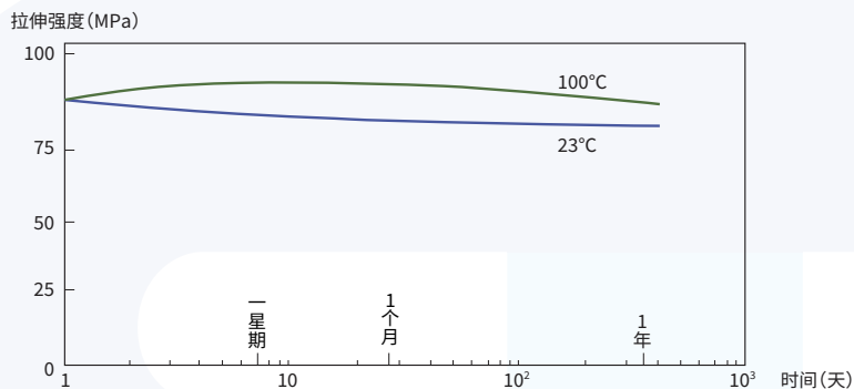
图3-1-5 水中拉伸强度的老化时间依赖性
