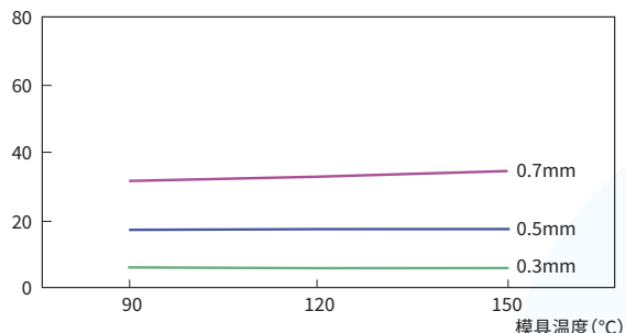
图4-2-16 模具温度依赖性(4100G)
