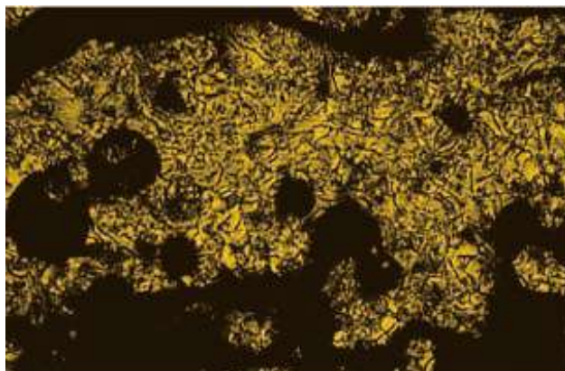
图1-1-5 SUMIKASUPER LCP 的偏光显微镜照片
