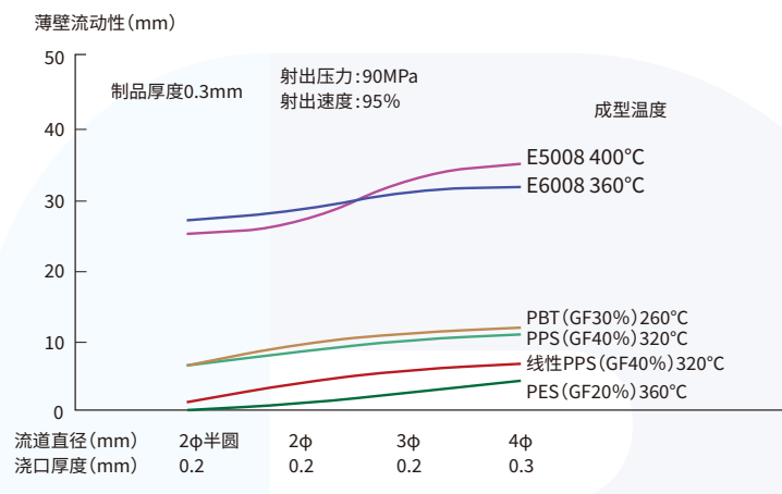
图4-3-6 薄壁流动长
