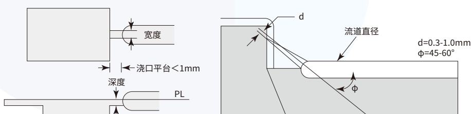
图4-3-7 浇口图
