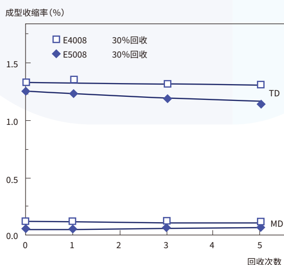
图4-4-2 回收次数与成型收缩率的关系
