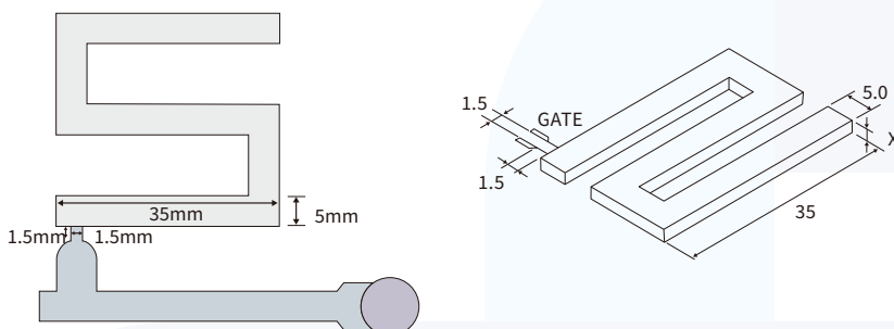
图4-2-7 薄壁流动长
