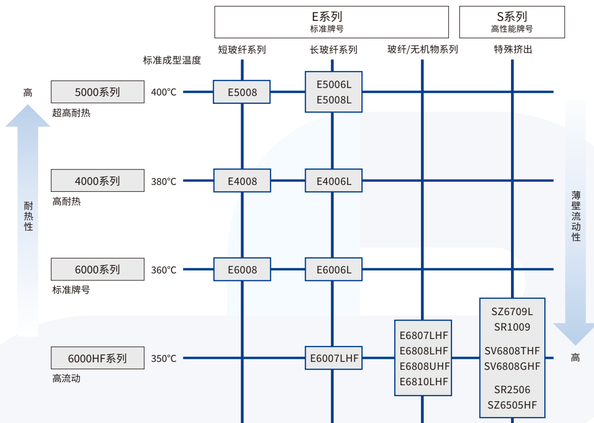
图1-2-1 SUMIKASUPER LCP 代表牌号的特征
