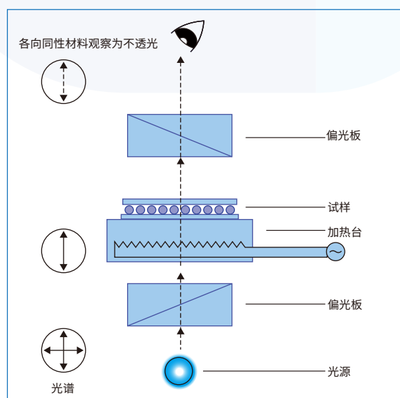
图1-1-3 熔融液晶观察装置
