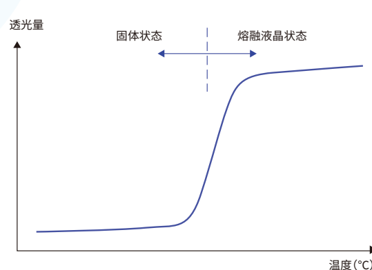
图1-1-4 温度与透光量的关系 (用偏光显微镜观察)
