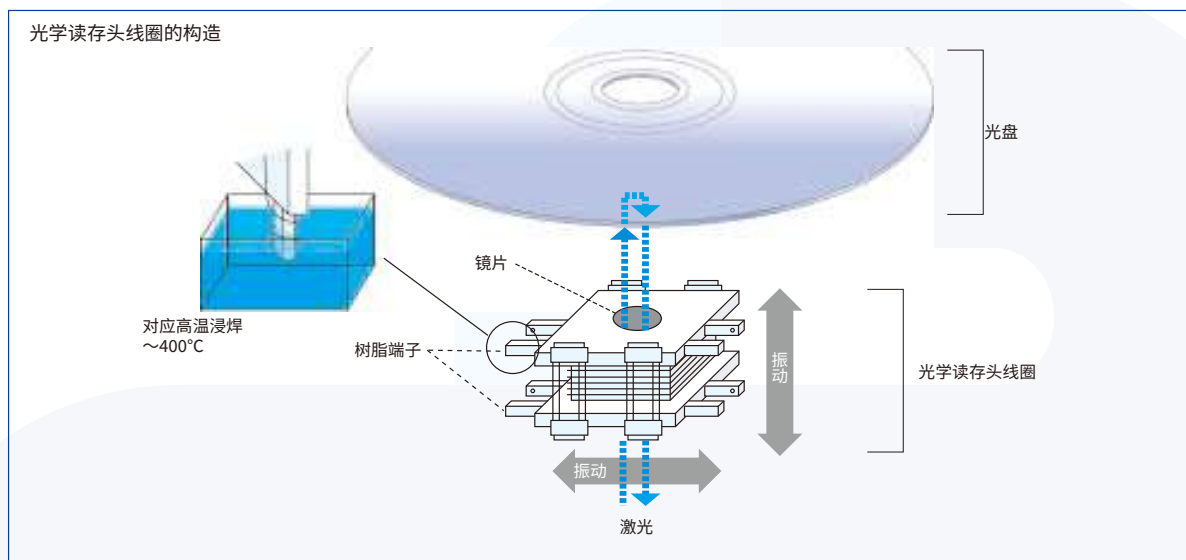
图6-3-1 光学读头线圈的构造
