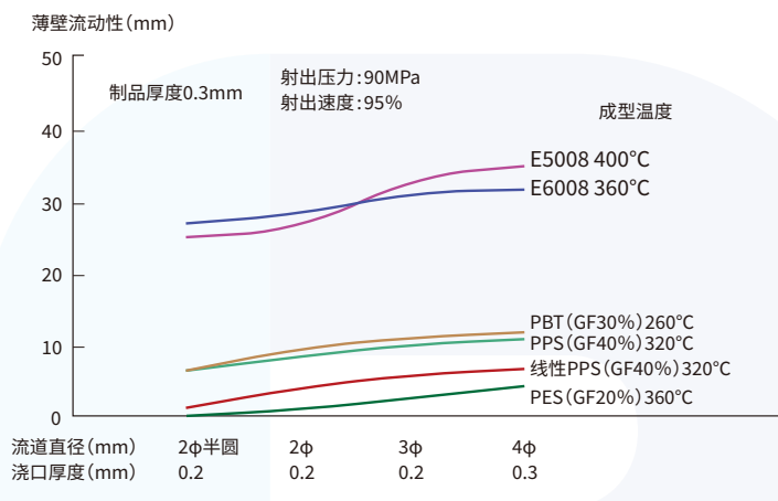
图4-3-6 薄壁流动长
