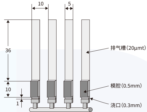
图4-1-4 飞边特性评价用模具
