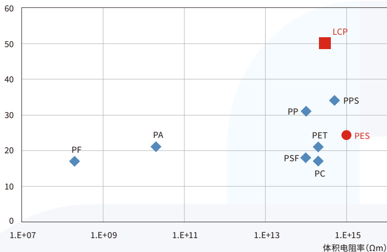
图3-6-1 SUMIKASUPER LCP 的体积电阻率与绝缘破坏强度
