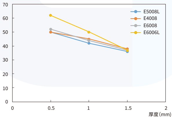
图3-6-2 SUMIKASUPER LCP 的绝缘破坏强度与厚度的依赖性
