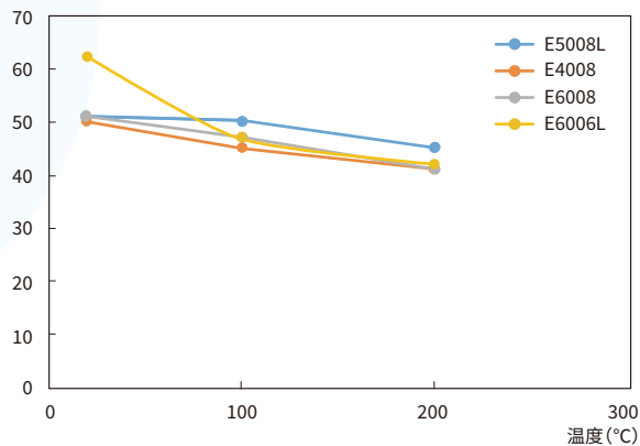
图3-6-3 SUMIKASUPER LCP 的绝缘破坏强度与温度的依赖性
