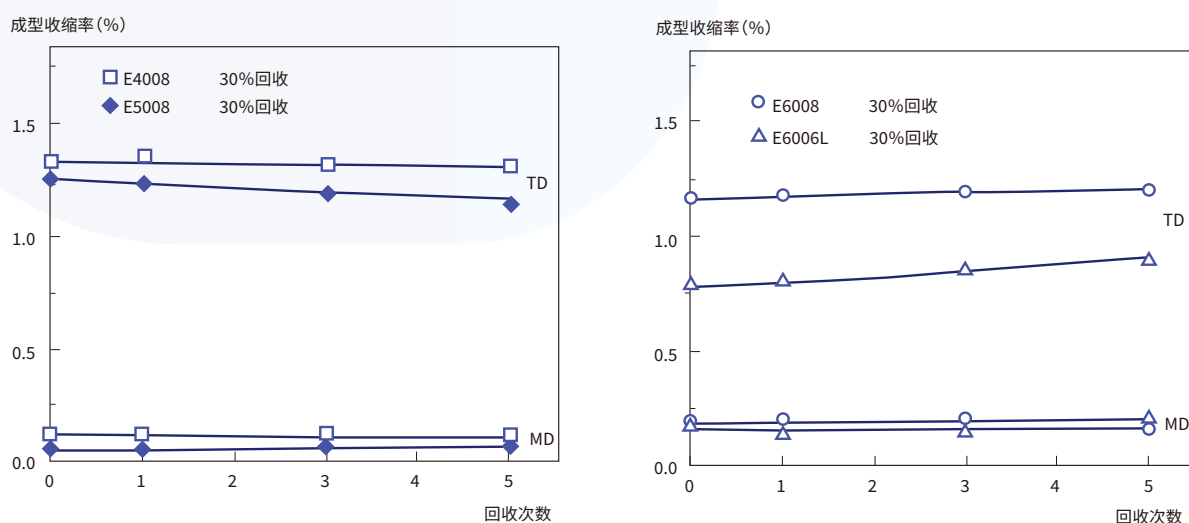
图4-4-2 回收次数与成型收缩率的关系
