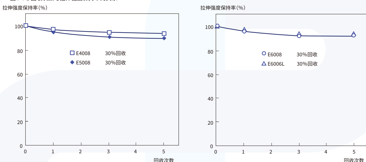
图4-4-1 回收次数与拉伸强度保持率的关系
