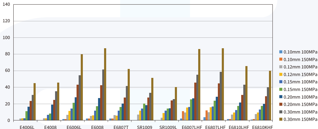
图6-2-3 SUMIKASUPER LCP 的薄壁流动性2
