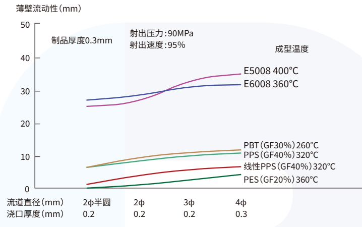
图4-3-6 薄壁流动长
