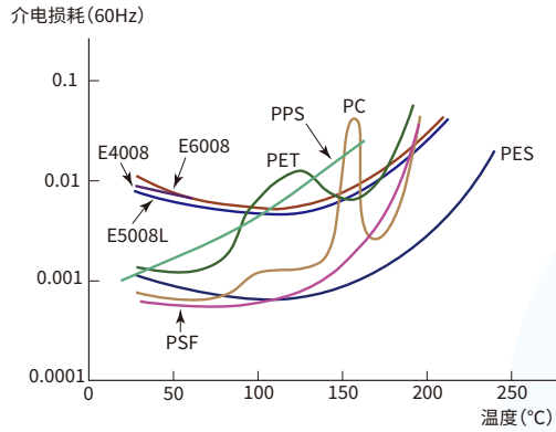
图3-6-4 介电损耗的温度依赖性
