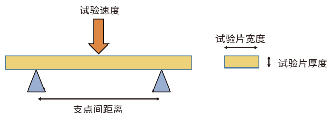
图6-2-4 薄壁强度测试试验方法
