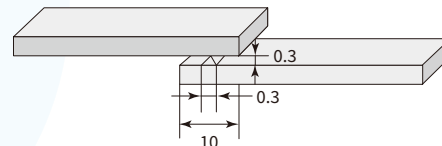
图5-2-1 超声波焊接的试验方法
