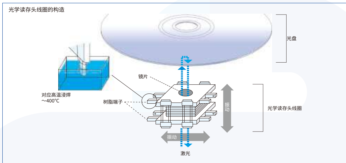
图6-3-1 光学读存头线圈的构造
