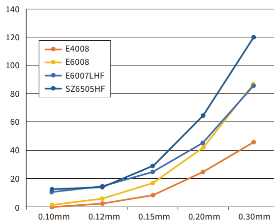
图4-2-9 薄壁流动长的厚度依赖性2
