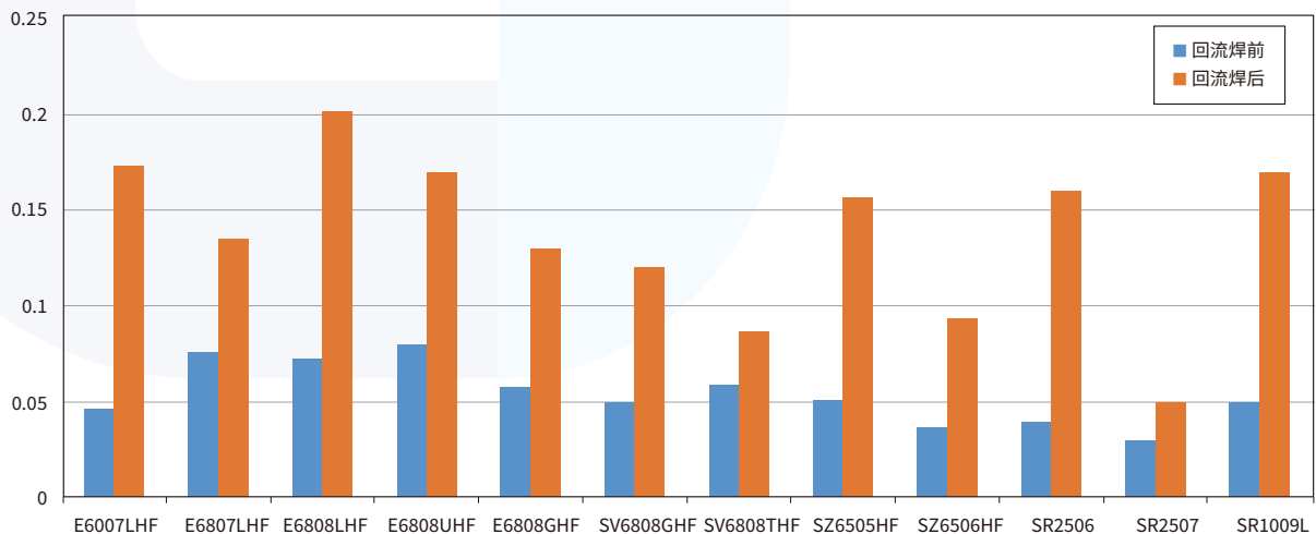
FPC模型连接器的翘曲量(mm)
