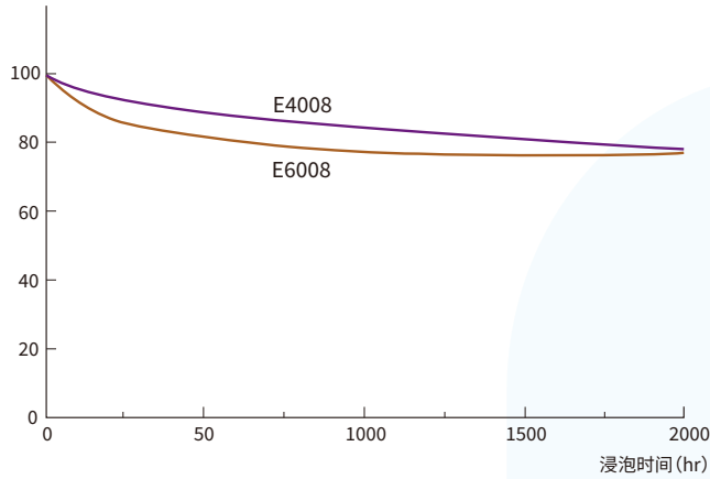
图3-1-4 SUMIKASUPER LCP 的耐热水性 (80℃)
