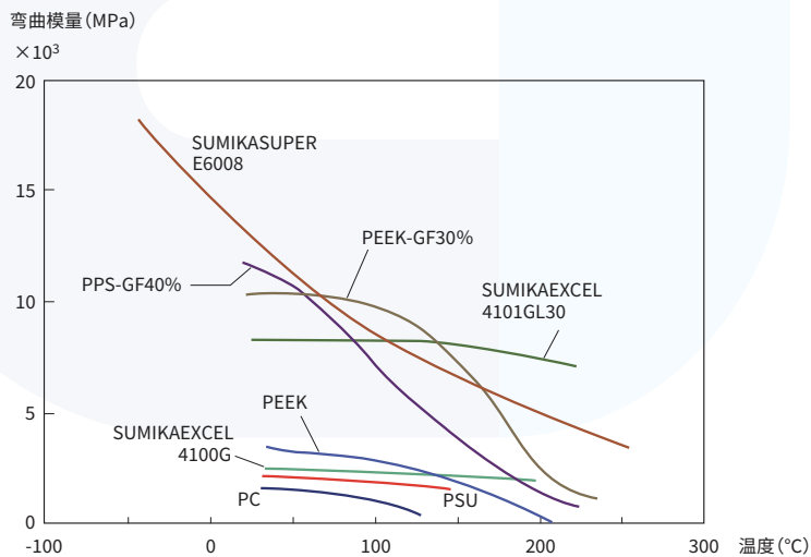
图3-2-3 弯曲模量的温度依赖性
