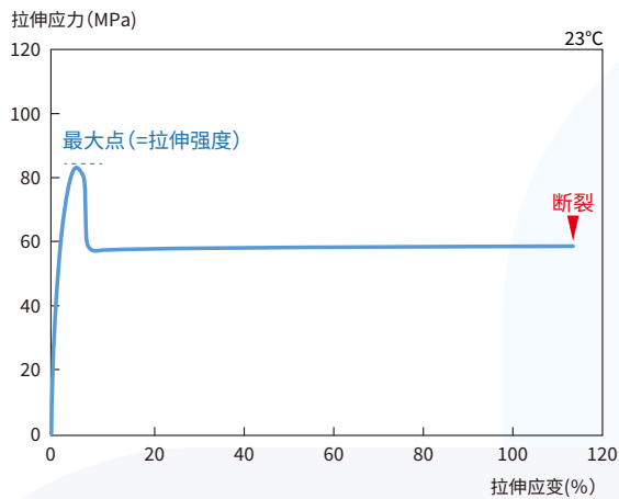
图3-2-1 4100G拉伸强度的S-S曲线
