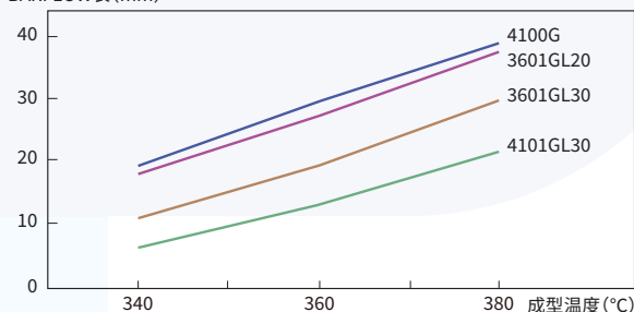
图4-2-8 机筒温度依赖性(0.5mm)
