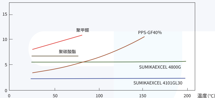
图3-3-2 线膨胀系数的温度依赖性
