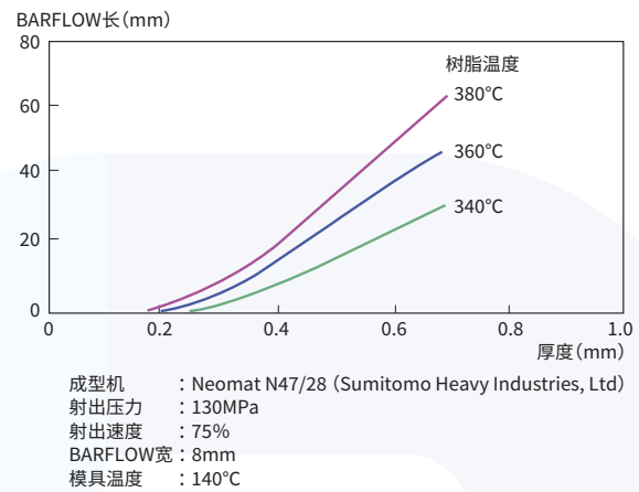
图4-2-11 厚度依赖性 (3601GL20)
