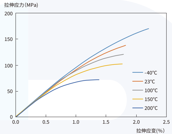
图3-2-2 4101GL30拉伸强度的S-S曲线
