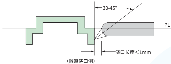
图4-3-4 点针式/隧道浇口形状
