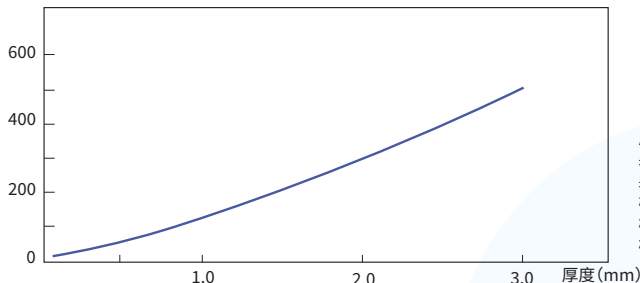
图4-2-6 BARFLOW长的厚度依赖性(4100G)
