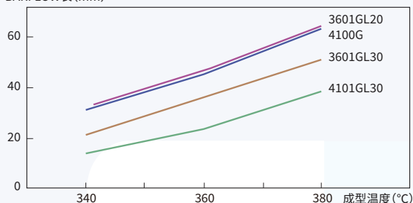
图4-2-7 机筒温度依赖性(0.7mm)
