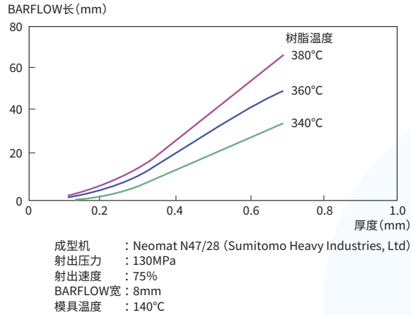
图4-2-10 厚度依赖性 (4100G)
