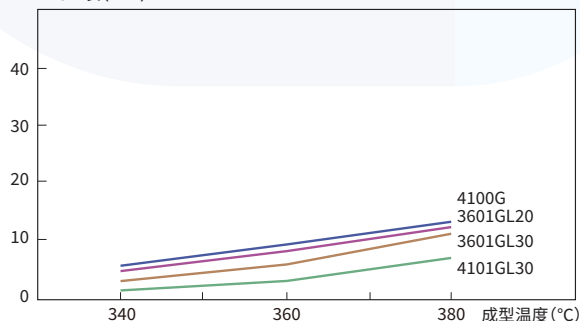
图4-2-9 机筒温度依赖性(0.3mm)
