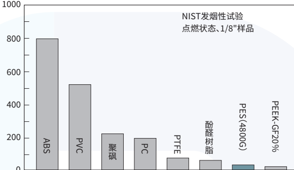
图3-4-2 发烟量
