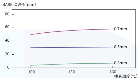
图4-2-17 模具温度依赖性(3601GL20)
