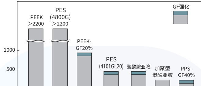
图3-2-4 SUMIKAEXCEL PES 的耐冲击性 悬臂梁冲击强度(3.2t,无缺口)(J/m)
