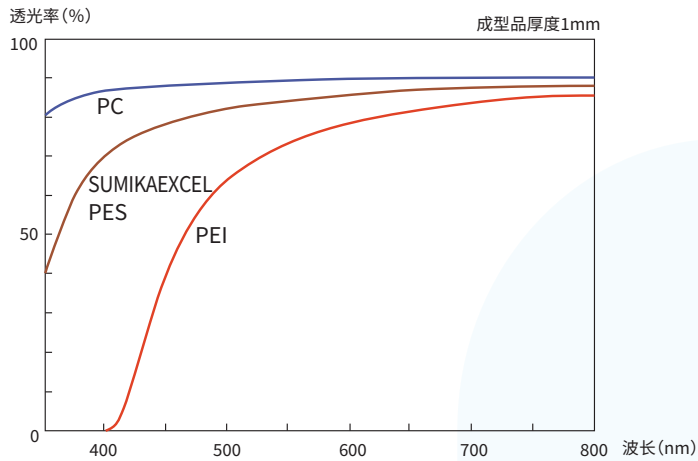
图1-1-3 SUMIKAEXCEL PES 的透光率
