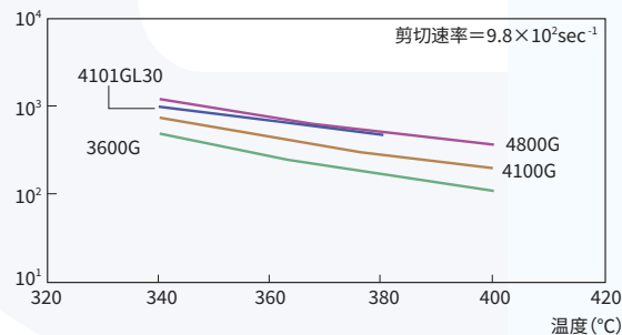
图4-2-1 表观熔融粘度的树脂温度依赖性
