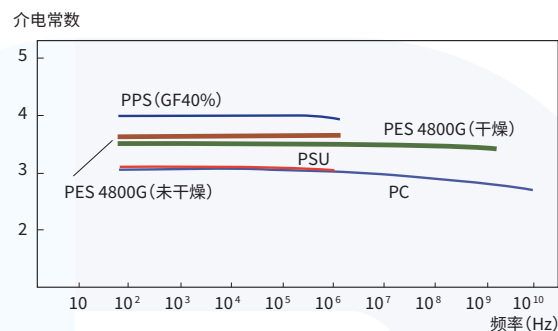
图3-6-2 介电常数的频率依赖性
