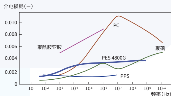
图3-6-4 介电损耗的频率依赖性(室温)
