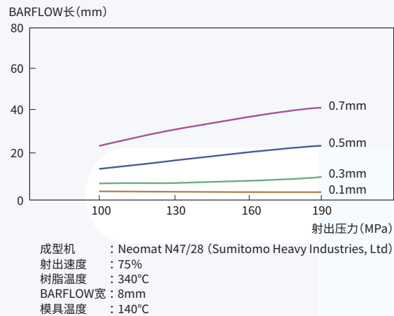
图4-2-12 射出压力依赖性 (4100G)
