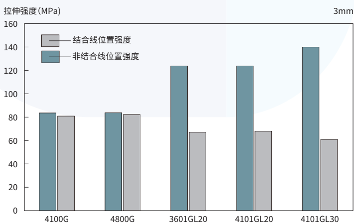
图3-2-7 拉伸强度
